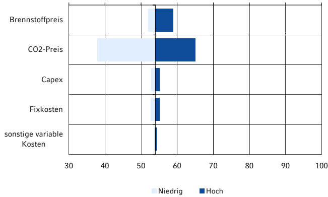
Stromgestehungskosten (€/MWh)
