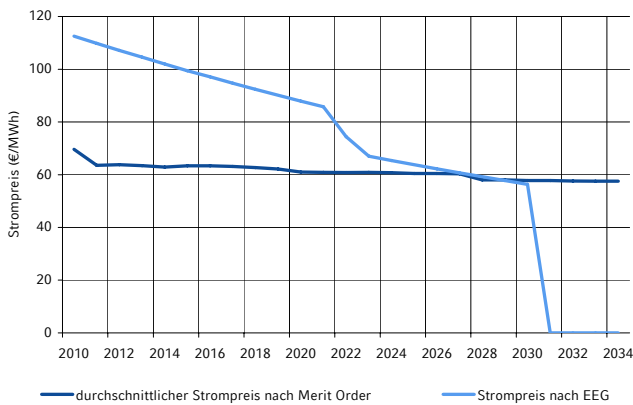
Onshore-Windkraft Großhandelsstrompreis unter Basisannahmen und Vergütung nach EEG (real)
