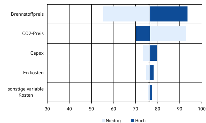
Stromgestehungskosten (€/MWh)
