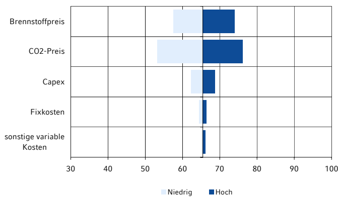
Stromgestehungskosten (€/MWh)
